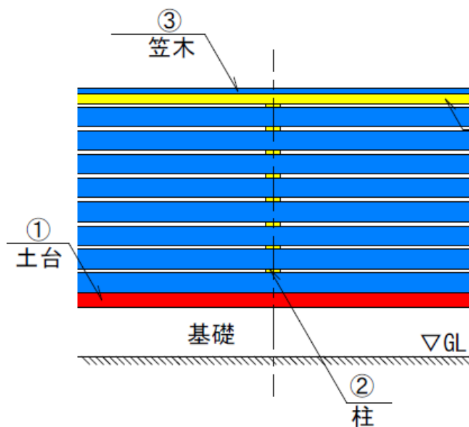
・塀（連続基礎・横板）の場合
