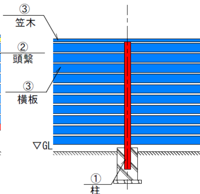
・塀（独立基礎・横板）の場合
