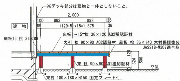
断面図 S=1/30 単位は mm
