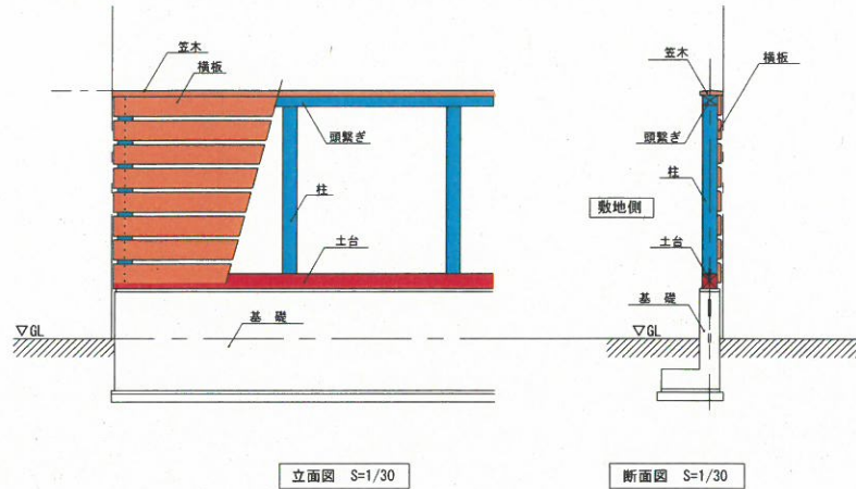
立面図 S=1/30
