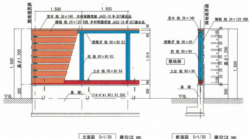
立面図 S=1/30 単位は mm
